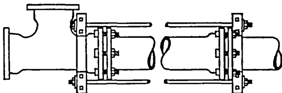
FIG. 96-13. TEE ANCHOR
