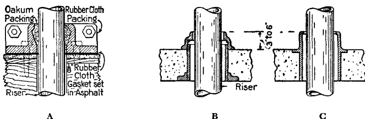
Fig. 480. Watertight Riser Sleeves.
