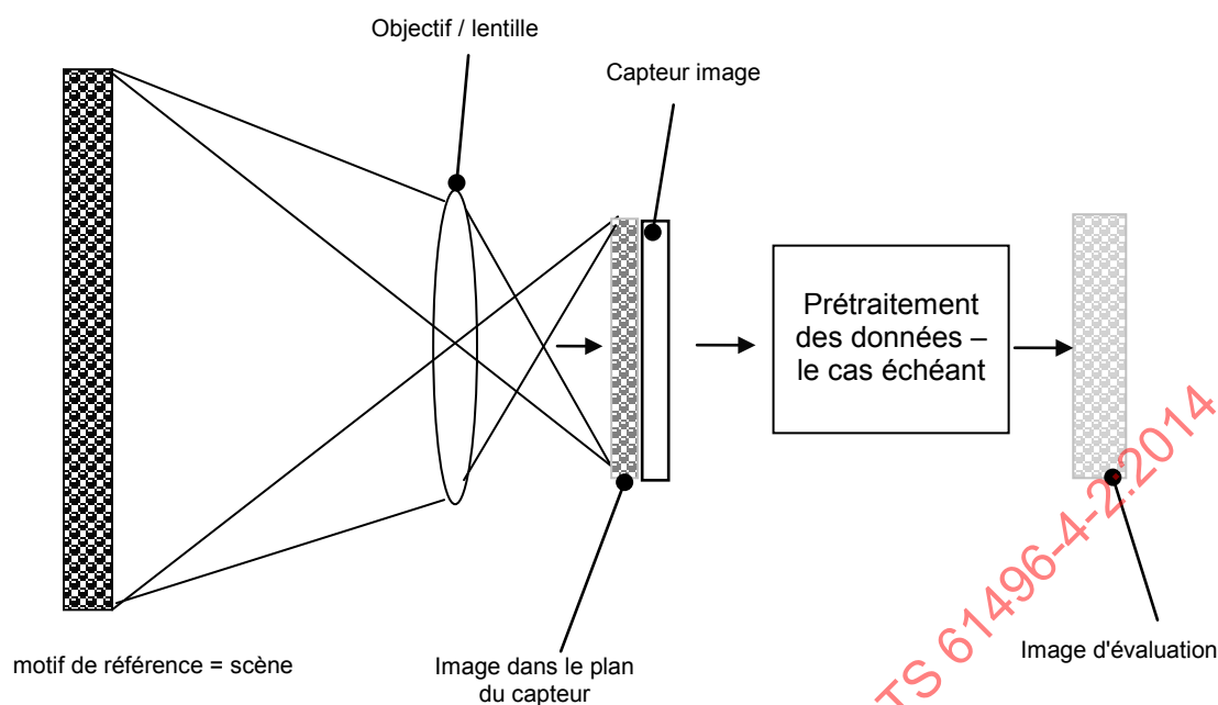
Figure 1 – Plans d'image avec le VBPDP
