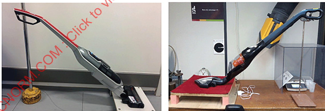
Figure 103 – Détermination du temps de fonctionnement du montage d'essai
