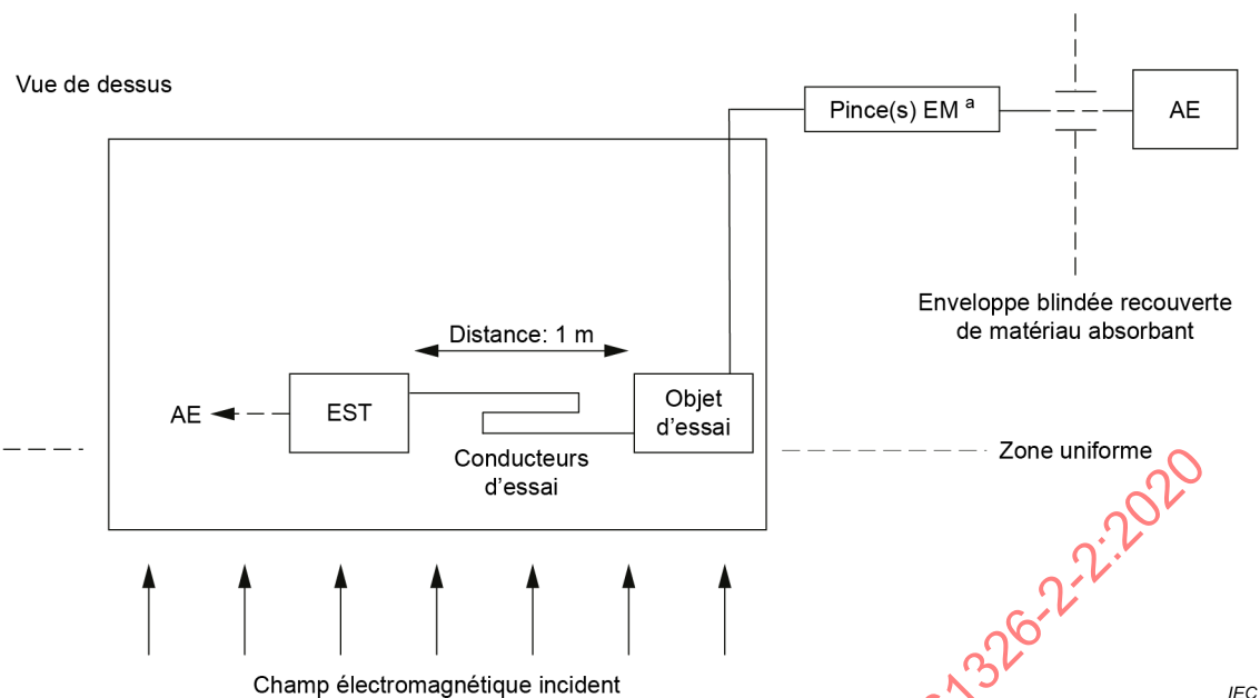
Figure 101 – Montage d'essai pour les matériels portables d'essai, de mesure et de surveillance fondé sur l'IEC 61000-4-3
