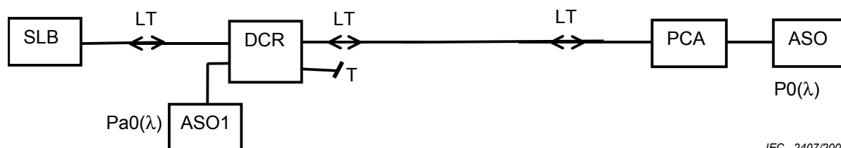
Figure 2 – Méthode à l'aide d'un analyseur de spectre optique – Etape 2
