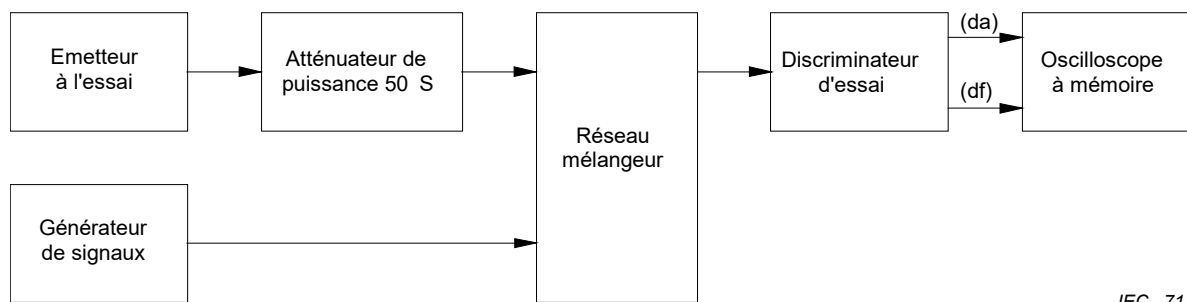
Figure 3 – Disposition pour l'essai de comportement aux changements de fréquences
