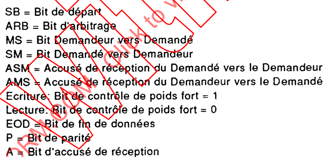
Figure 6 - Format de la trame
