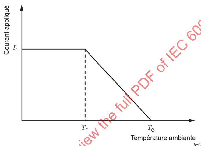
Figure 1 – Relation entre la température ambiante et le courant appliqué
