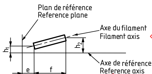
Figure 5 - Décalage permis de l'axe du filament 9) Permissible offset of filament axis 9) (Seulement pour lampes étalon/For standard lamps only)
