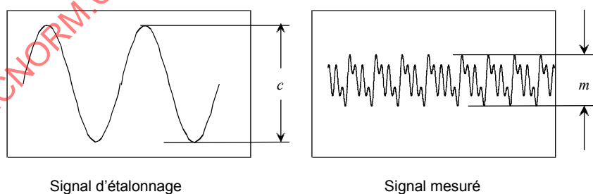
Figure 7 – Affichage sur l'oscilloscope
