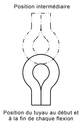
Figure 105 – Positions de flexion pour le tuyau après retrait de l'armoire de congélation
