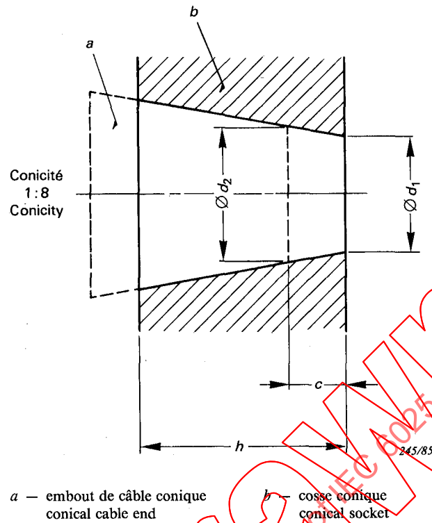
FIG. 1. — Dimensions de base des bornes coniques terminales des batteries de traction. Basic dimensions of conical traction battery terminals.
