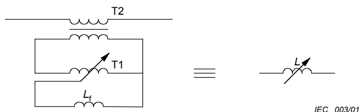
Figure 3 – Montage pour réaliser la bobine d'inductance variable L de la figure 2
