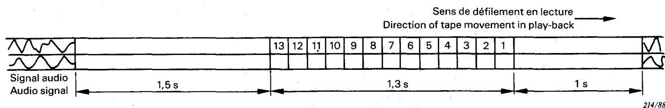
FIG. 2b. — Position des impulsions sur la bande. Position of the pulses on the tape.
