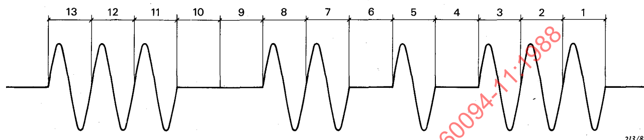
FIG. 1. — Exemple de signal de code. Example of a code signal.
