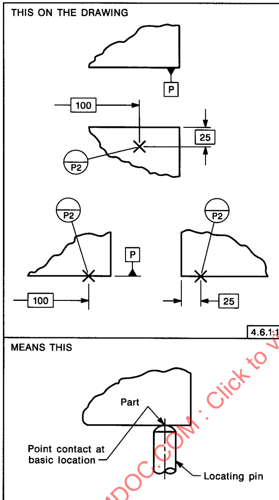
FIG. 4-27 DATUM TARGET POINT
