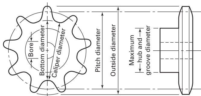
Fig. 7 Sprocket Diameters
